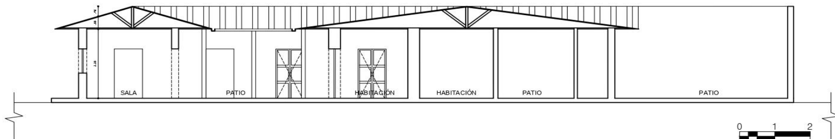
Corte longitudinal
